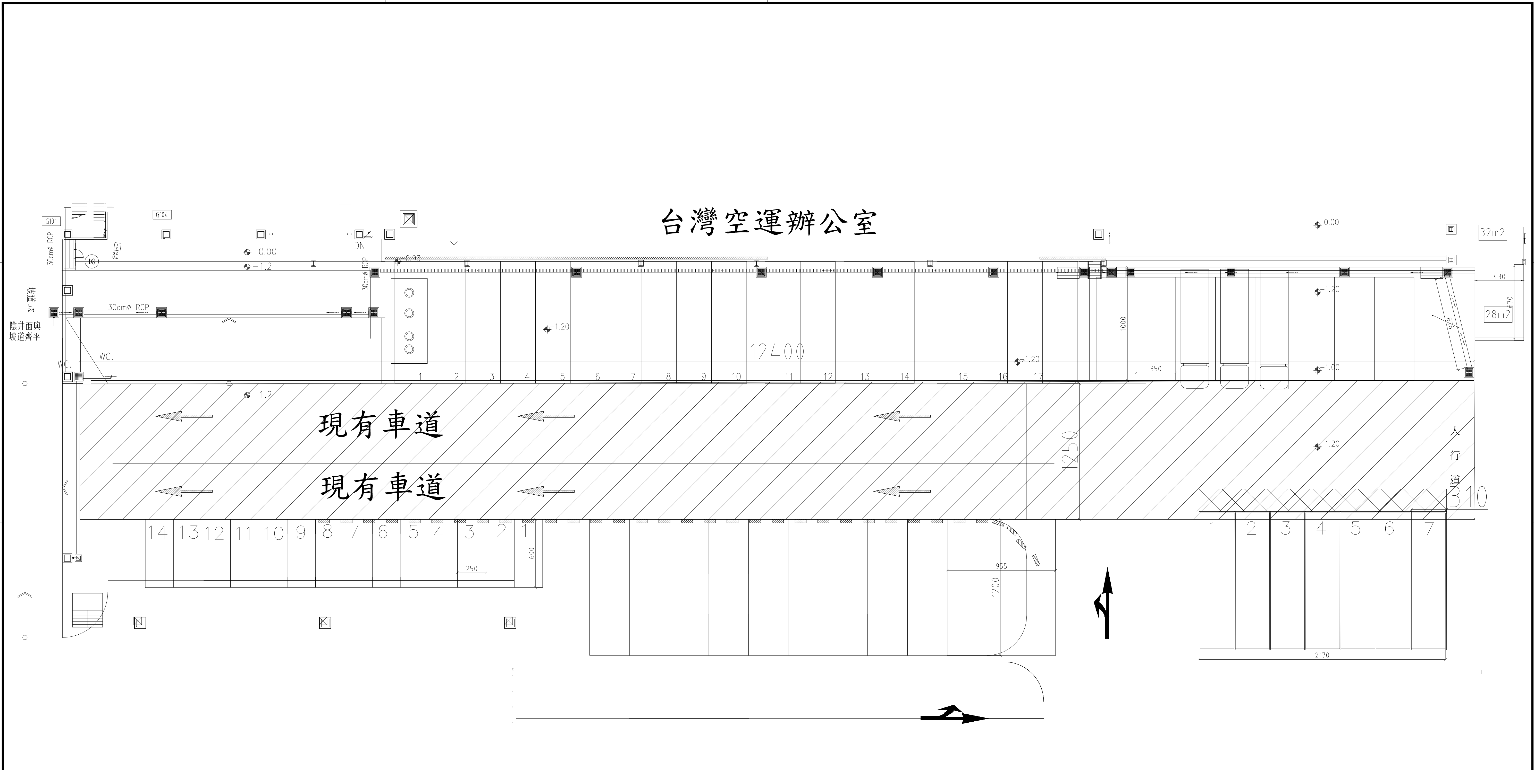
進口倉陸側S庫至25號通道前車道洩水改善工程示意圖
